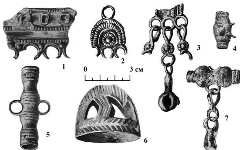
Рис. 1. Находки М. С. Знаменского с городища Искер. Материал: 1-7 – бронза
