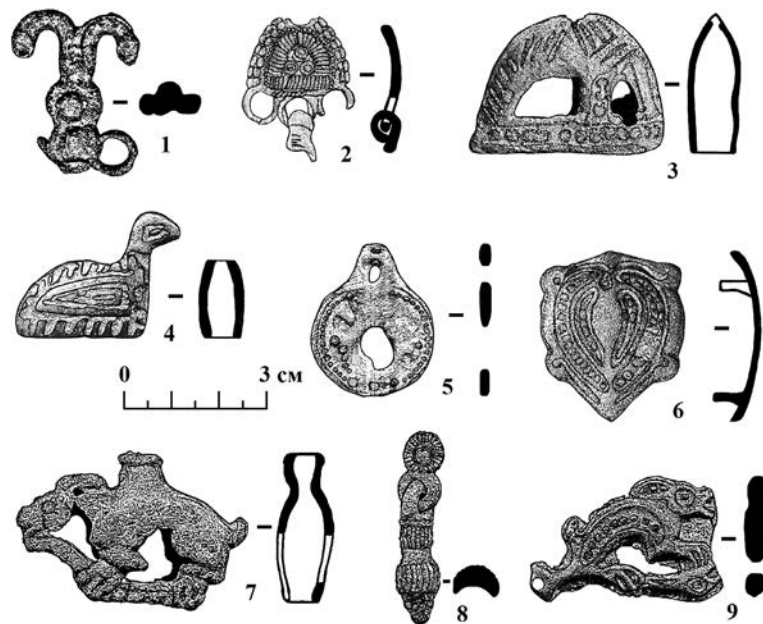
Рис. 2. Городище Искер. Предметы металлопластики. Материал: 1-9 – бронза
